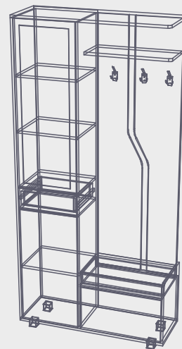
КМ.343.001 Размеры: 1000x2097x353
